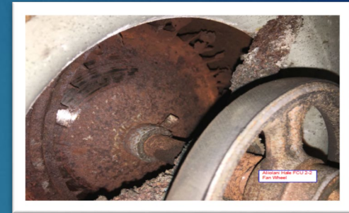
Fan Wheel
